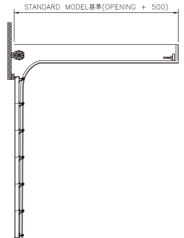
C-30 立面図
